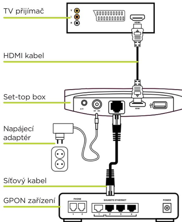
Obr. 3: Propojení set-top boxu s televizorem pomocí HDMI kabelu.
