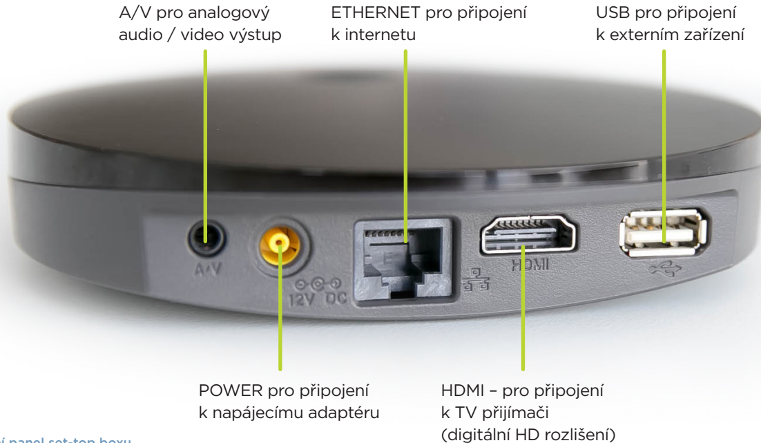
Obr. 2: Zadní panel set-top boxu
