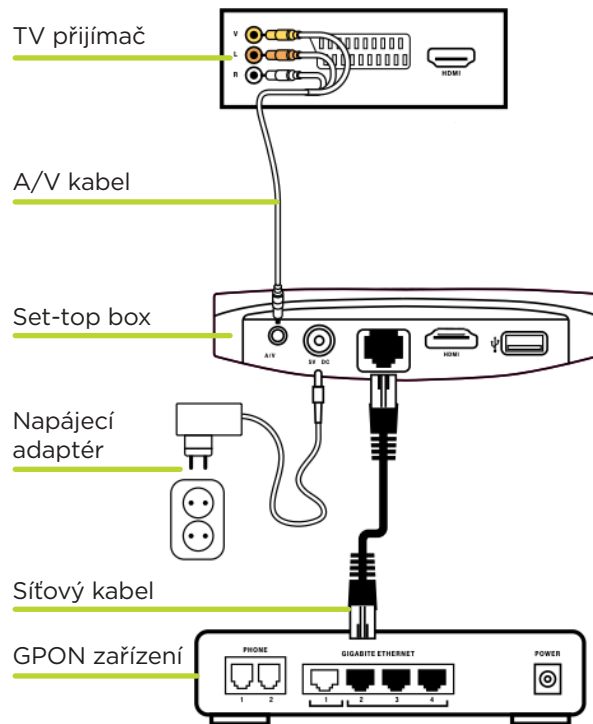
Obr. 4: Propojení set-top boxu s televizorem pomocí kabelu jack.
